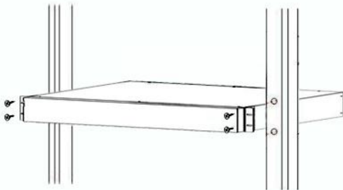
图2-2 安装设备到机柜中
