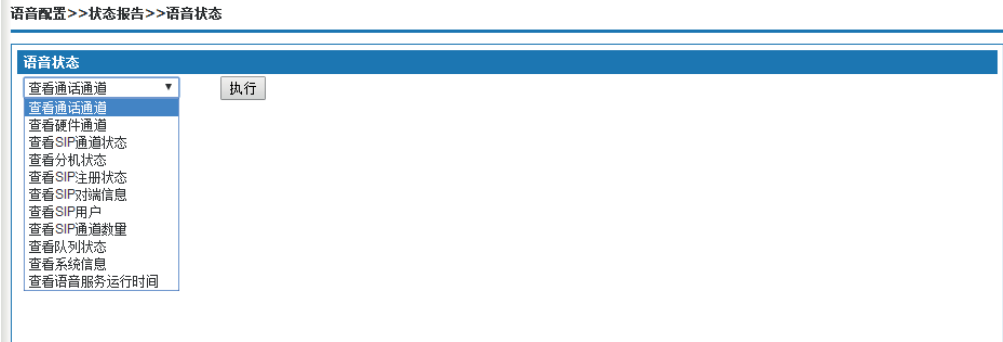
图6-135 语音状态
