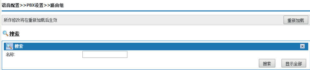
图6-118 路由组-搜索
