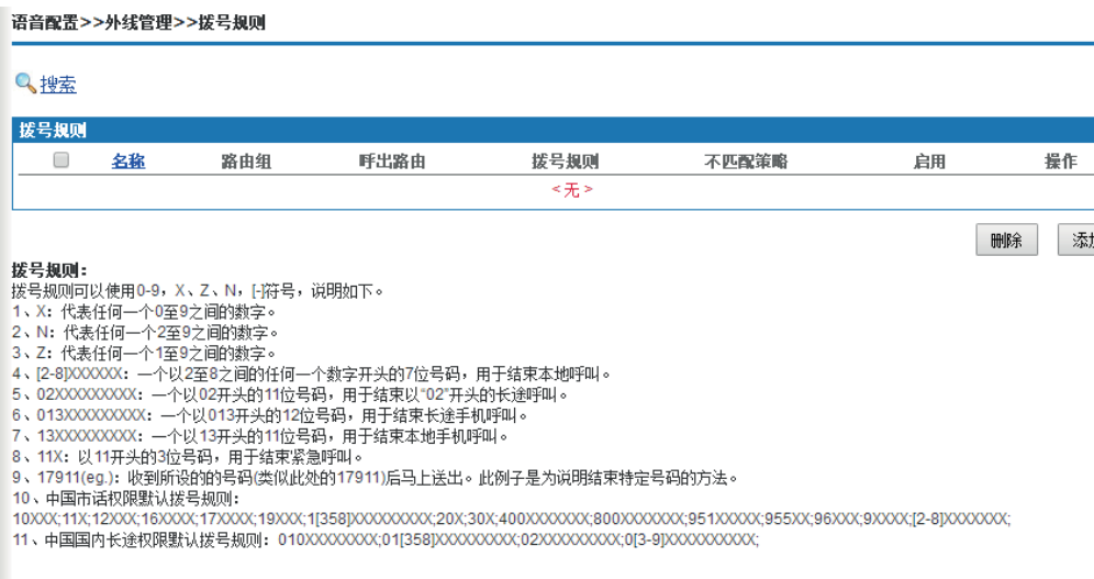
图6-49 拨号规则
