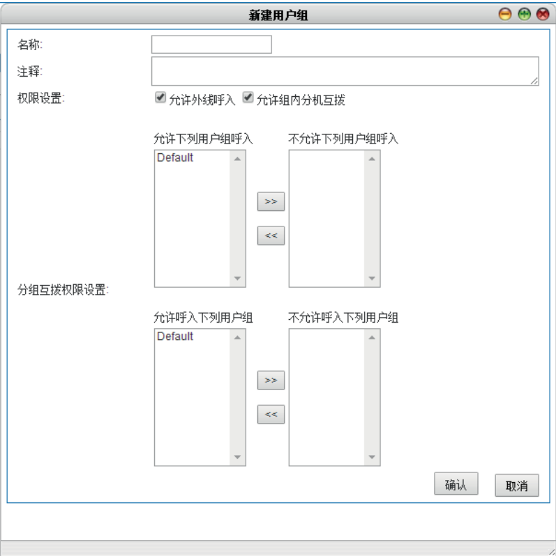
图6-21 新建用户组
