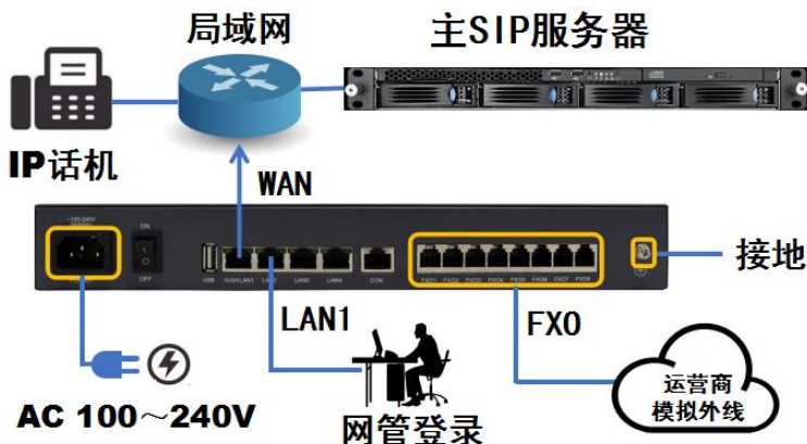
图3-1 连接HB IP PBX和终端PC
