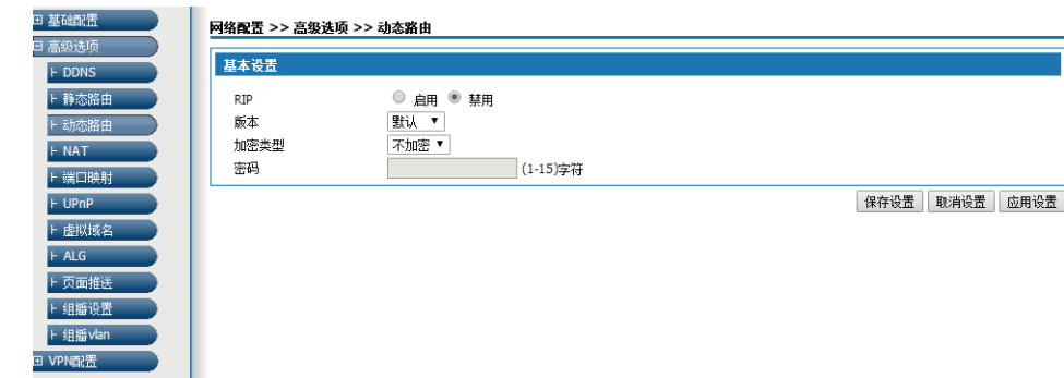
图5-14 动态路由
