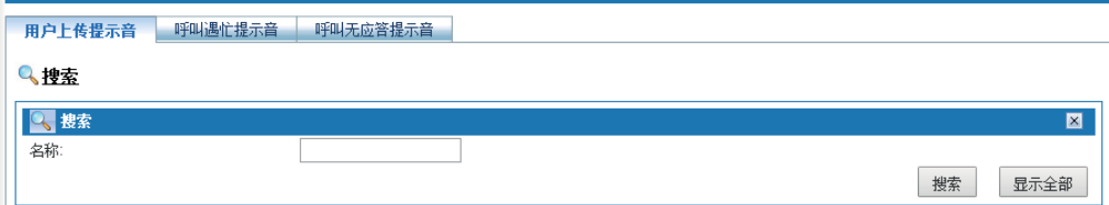
图6-121 搜索提示音
