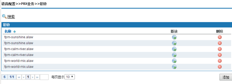
图6-73 彩铃
