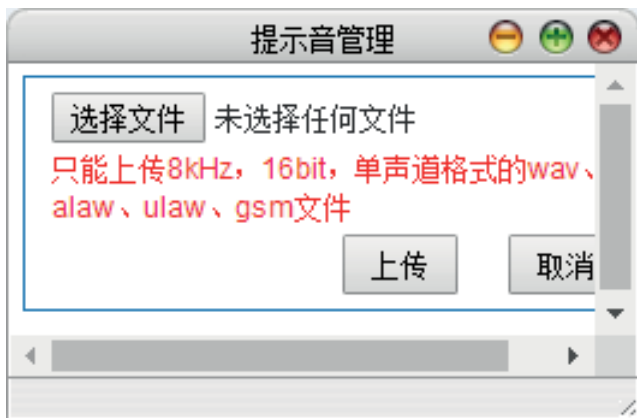
图6-120 添加提示音
