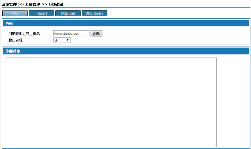
图10-13 系统调试
