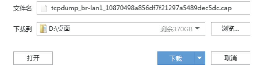
图6-137 数据包保存
