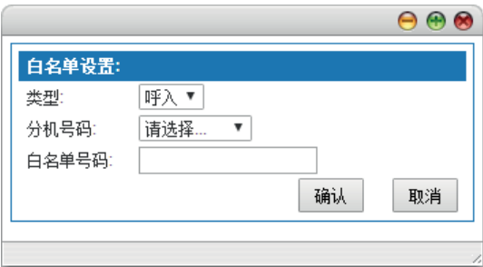
图6-90 添加白名单
