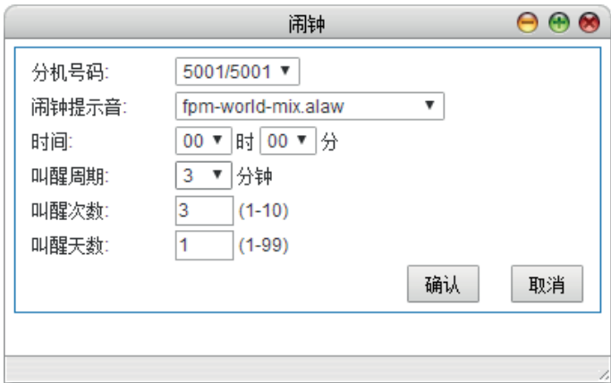
图6-77 添加闹钟
