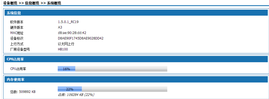
图4-1 系统概览
