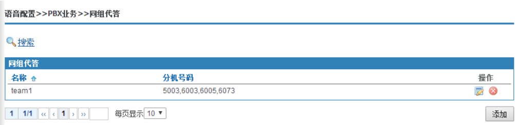
图6-70 同组代答
