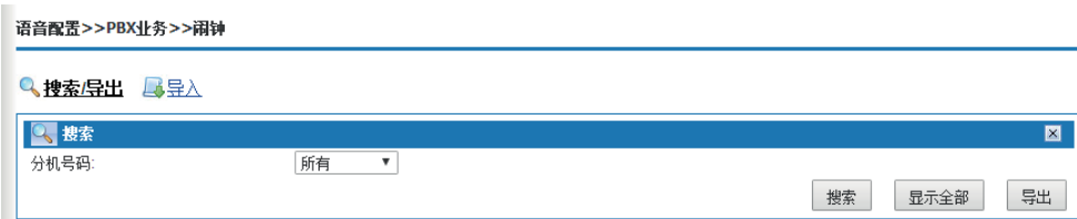
图6-78 搜索闹钟用
