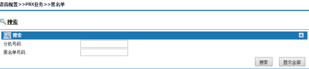
图6-88 搜索黑名单
